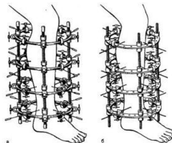
Рис. 79. Аппарат Калнберза: А – скелетно-мышечный, Б – операционный.
